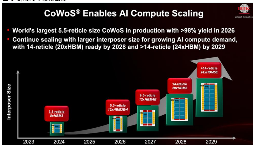
圖 1: 封裝尺寸擴張路徑
